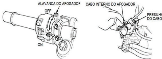
ALAVANCA DO AFOGADOR CABO INTERNO DO AFOGADOR
