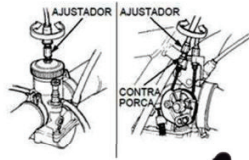
CONTRAPORCA AJUSTADOR
